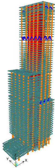
Fig. 3 Setback elevation
