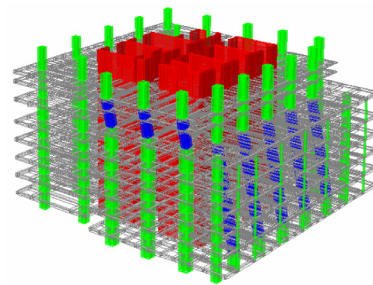
Fig. 4 Inclined columns
