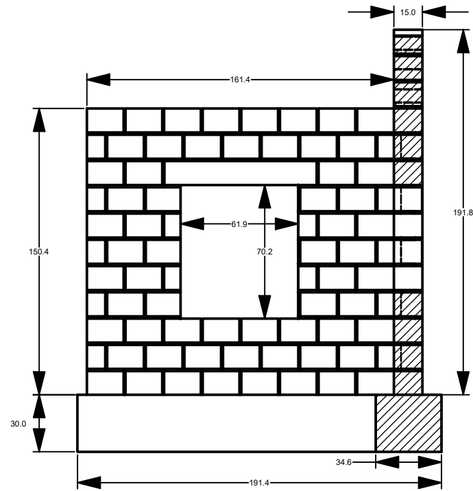
Section A-A Scale 1:1
