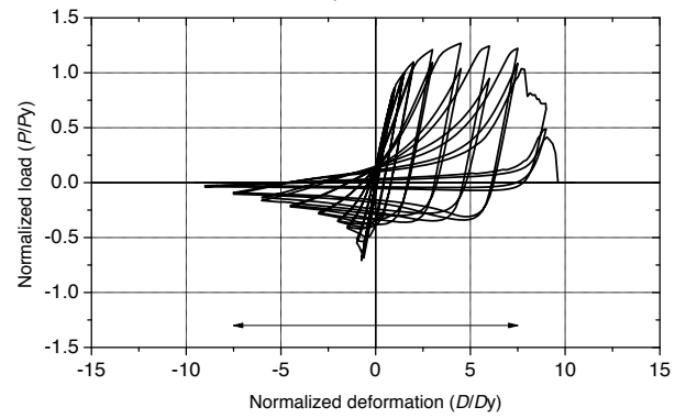
(d) KL/r = 100
