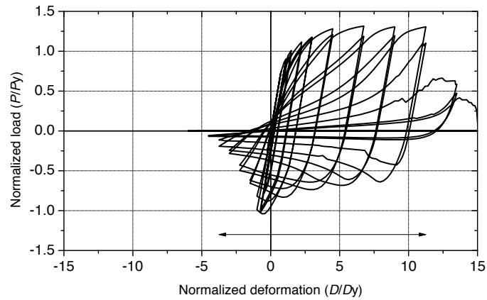
(c) tension:compression=3:1
