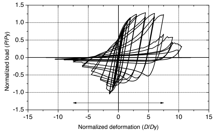
(b) tension:compression=1:1
