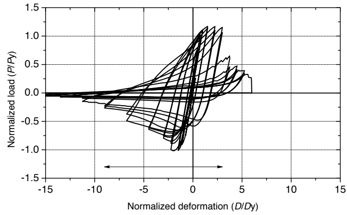
(a) tension:compression=1:3
